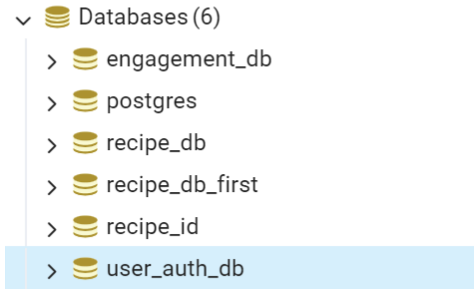
Рисунок 1 – Разделенные БД
