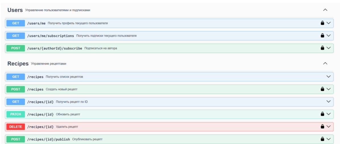
Рисунок 2 – SwaggerUI
